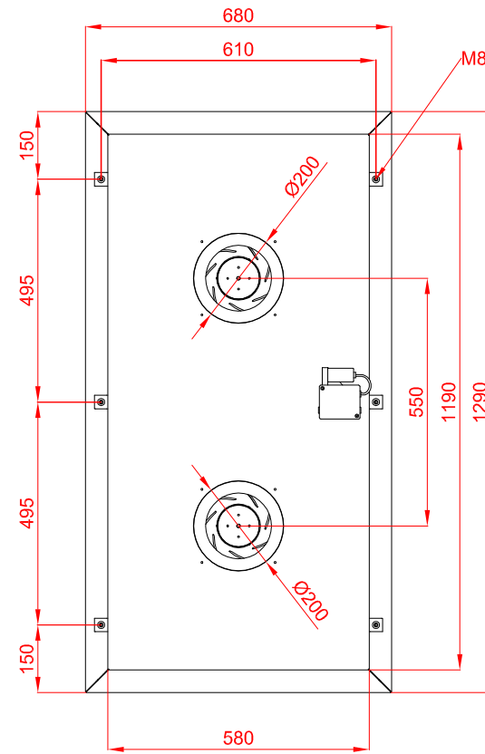
DIFVENT 6/12
